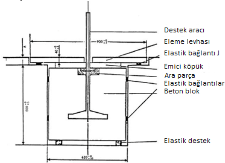
Şekil 10.3 Deney cihazı
